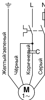
Рис. 13 Электродвигатели фирмы Franklin
