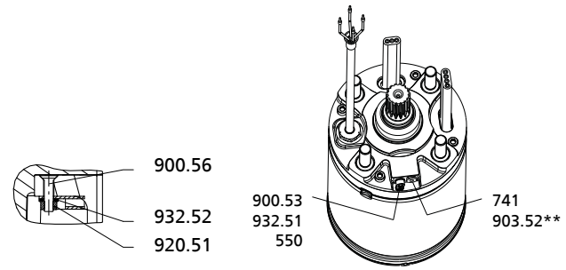
Крепление заземления
