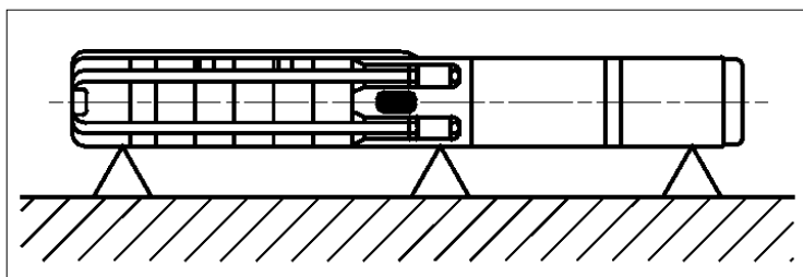
Рисунок 6 - Способ хранения на опорах
