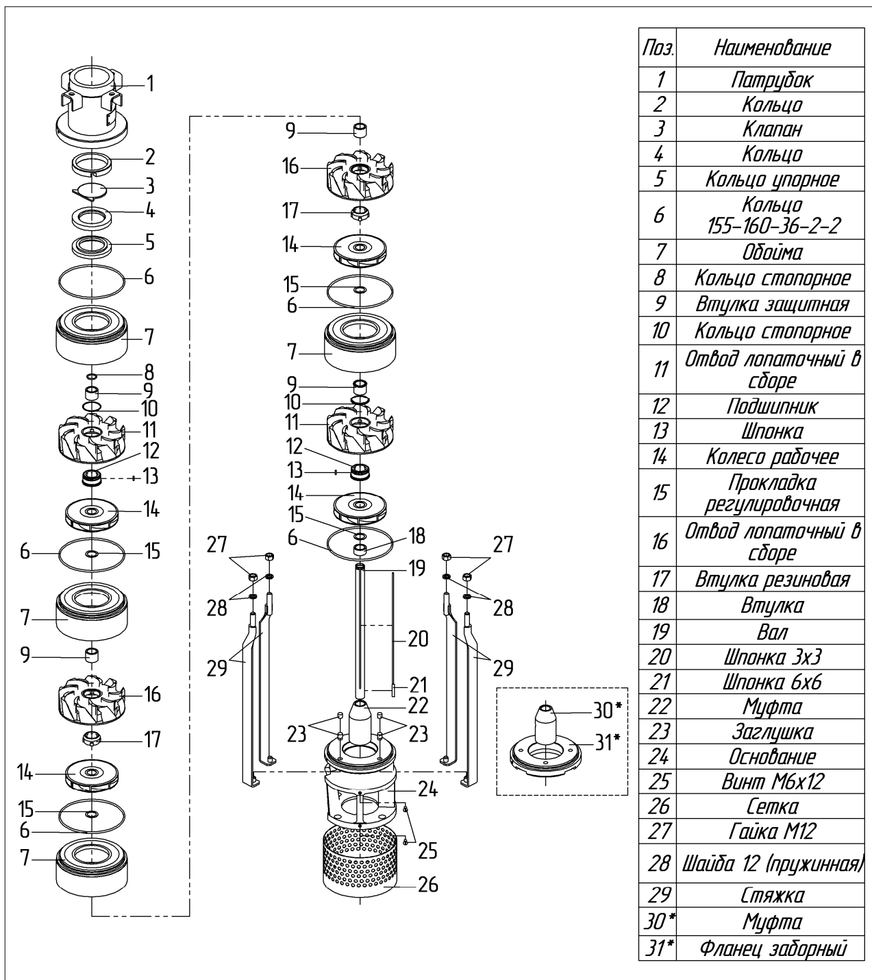
Схема разборки насоса ЭЦВ 8-40 (комплектация электродвигателем ДАП)
