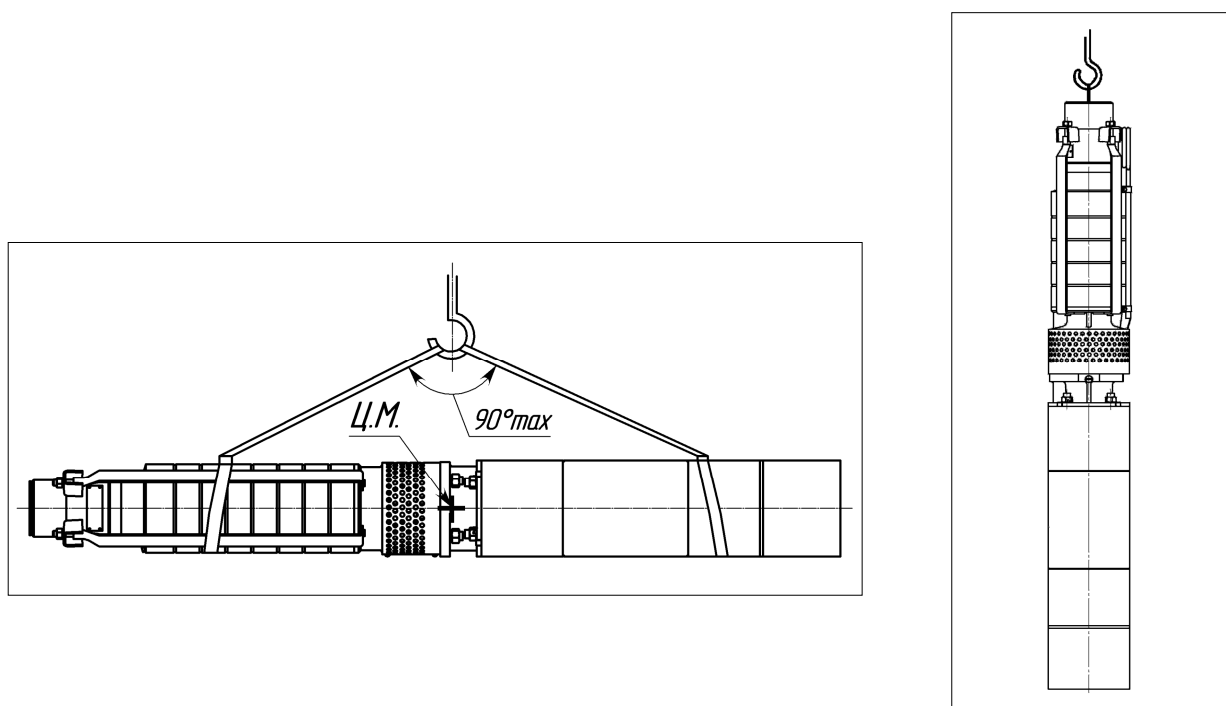
Рисунок 7 – Схемы строповки
