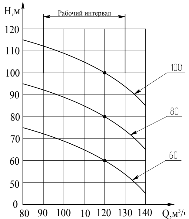
2ЭЦВ 12-160 и ЭЦВ 12-160
