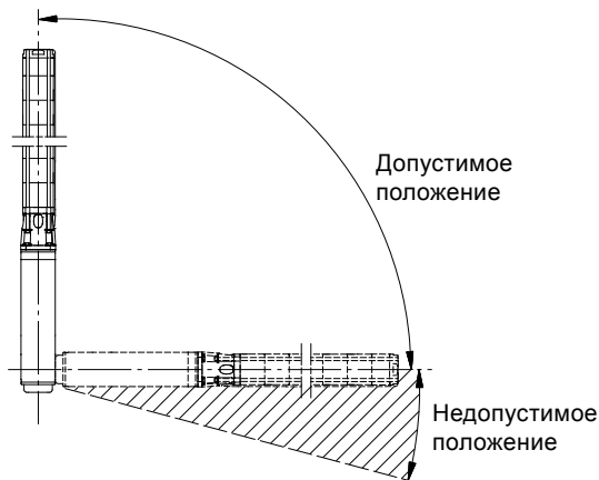
Рис. 8 Монтаж
