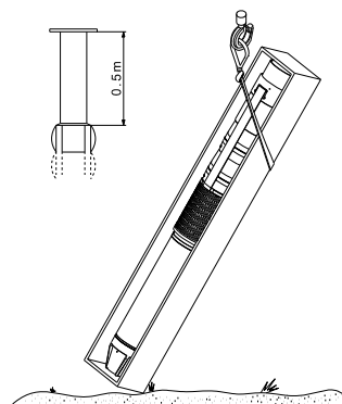
Рис. 19 Подъем и установка насоса в вертикальное положение
