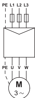
Рис. 15 Электродвигатели Grundfos - прямой пуск
